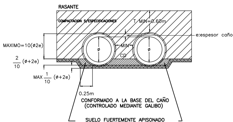
ESCALA 1:25
