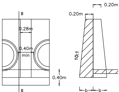
SEMICORTE I-I
