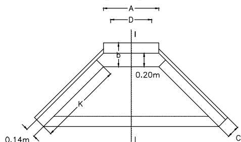
SEMI-PLANTA
