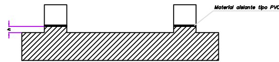
CORTE A-A
