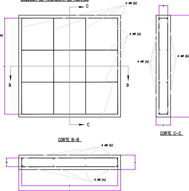
ESQUEMA DE ARMADURA DE HIERROS
