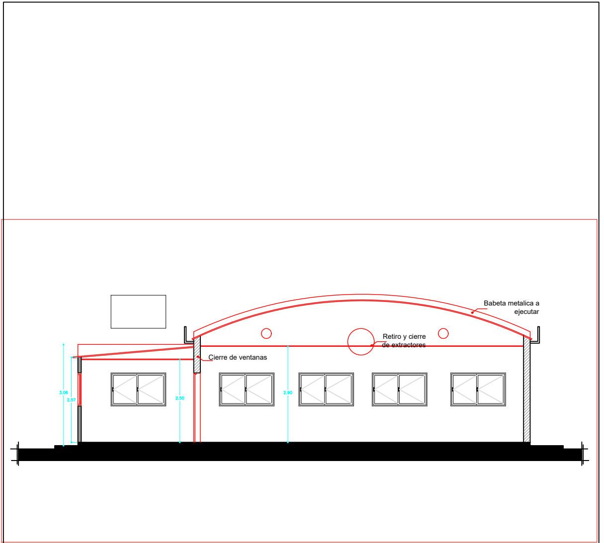
CORTE A-A - ESC 1:100
