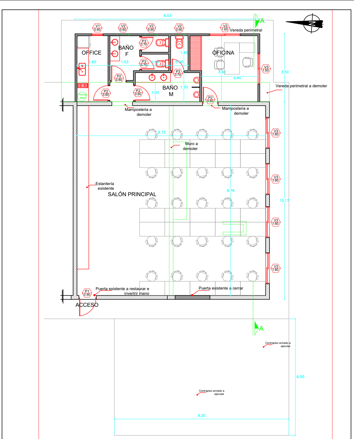
PLANTA - ESC 1:100
